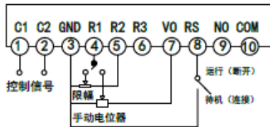
图 6：手动与限幅功能的自动控制接线图
